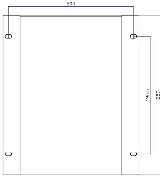
主视图
